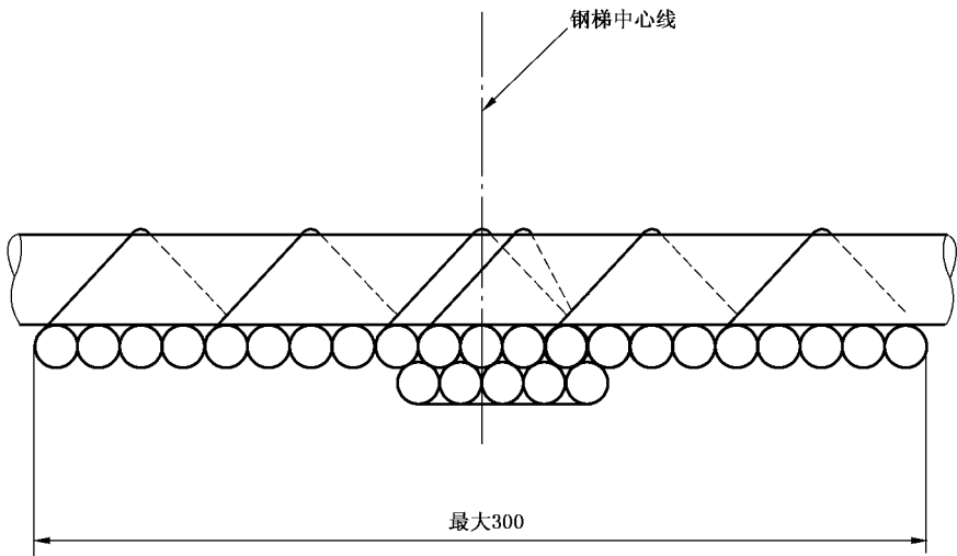
图 1 接触安装在标准钢梯前面的电缆(相互接触的电缆试样段组)
