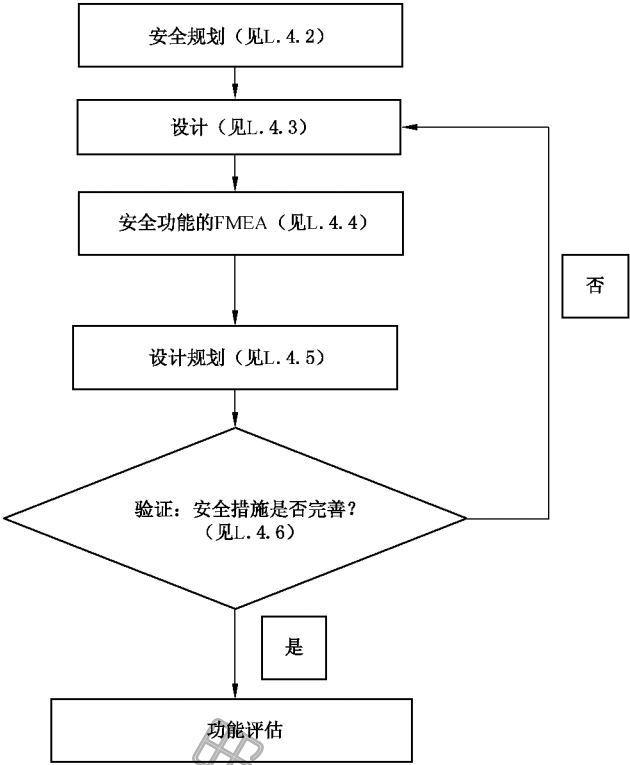
图 L.1 安全设计流程
