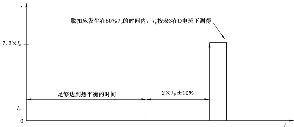
图 2 热记忆试验
