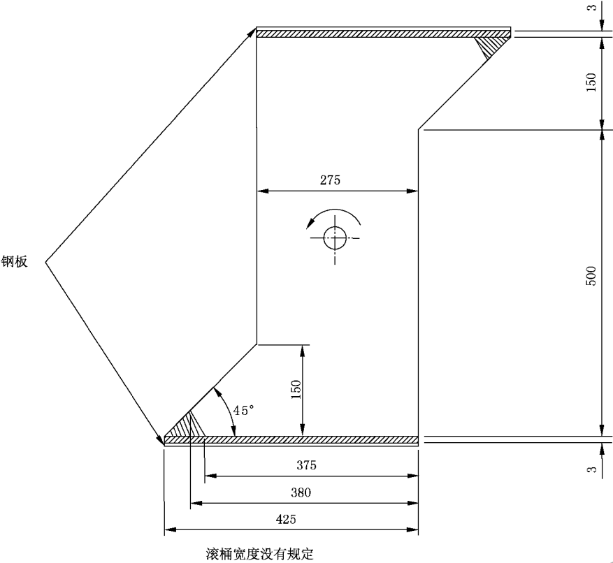
图 25 滚桶
