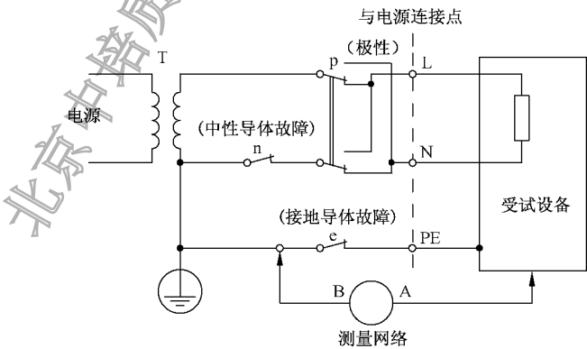
图 G.1 在星形 TN 或 TT 系统上的单相设备的试验配置
