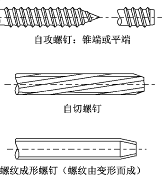
图 22 自攻螺钉、自切螺钉和螺纹成形螺钉的例子
