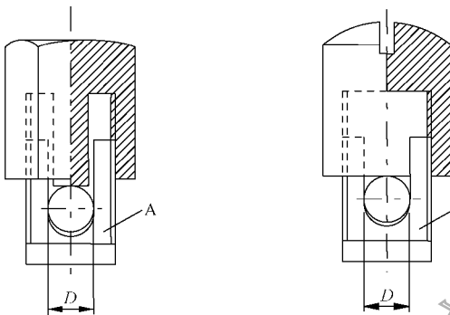
图 15 接片接线端子
