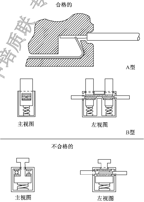
图 17 电气连接件结构图
