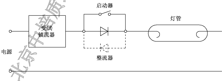
图 C.2 整流效应的试验线路(单脚灯管的镇流器)
