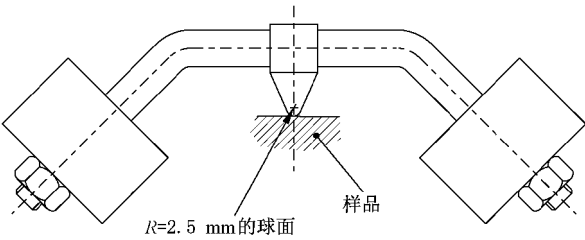
图 10 球压装置
