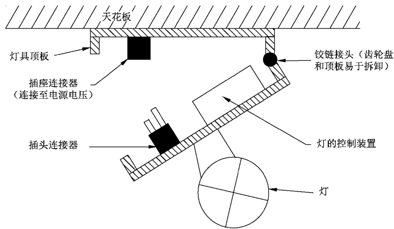
图 31 插头/插座连接的电气-机械接触系统
