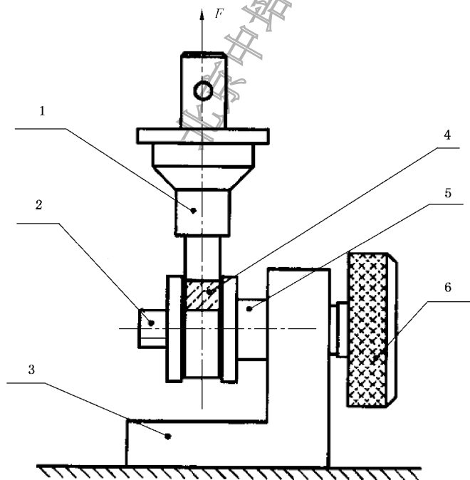
图 A.1 管环转盘支架示意图
