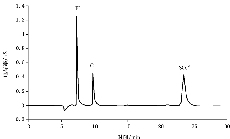
图3 阴离子交换柱分离效果图
