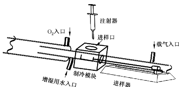
图2 舟进样系统结构
