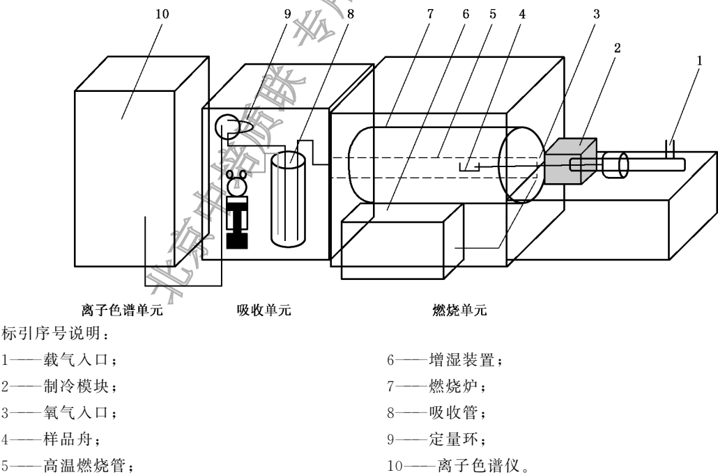
图 1 燃烧-离子色谱仪结构示意图
