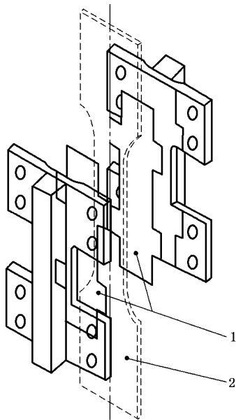
图 10 板状试样的夹持示意图
