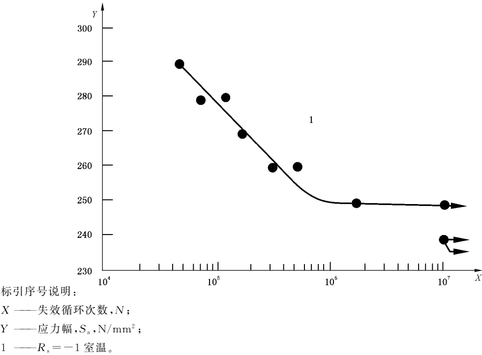
图 3 Wöhler 曲线或 S-N 曲线
