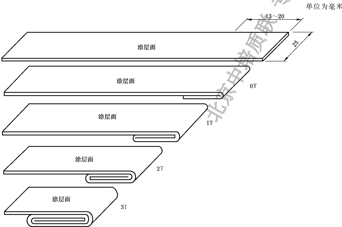
图 1 T 弯过程示意图
