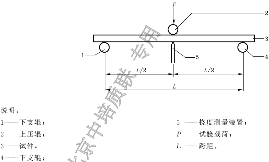
图 3 弯曲装置及试验示意图
