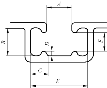
图 C.2 浇注型材槽口示意图
