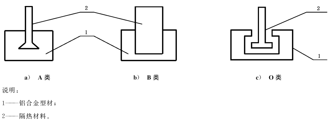
图 2 隔热型材的剪切失效类型
