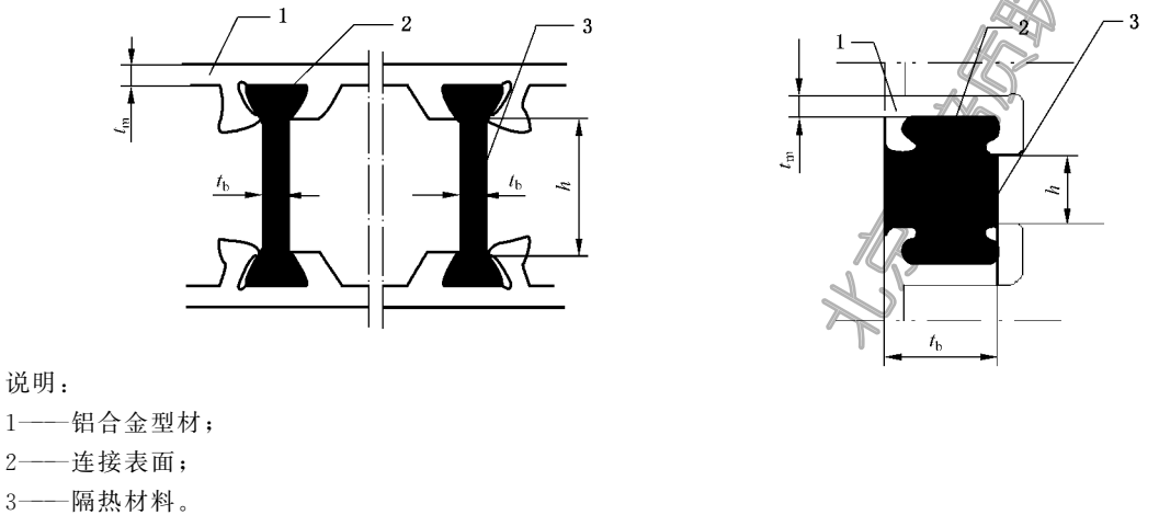
图 B.1 铝合金型材与隔热材料连接示意图
