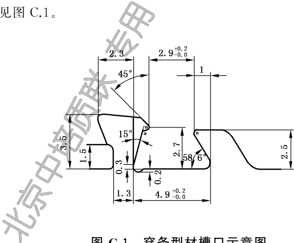
图 C.1 穿条型材槽口示意图
