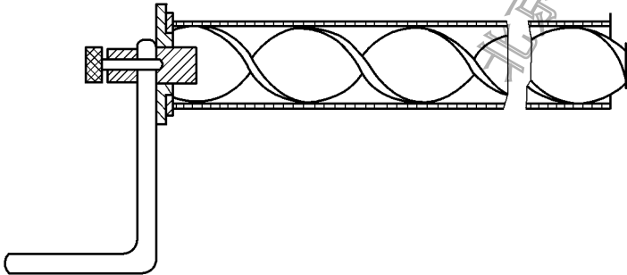
图 2 e) 手工螺旋钻
