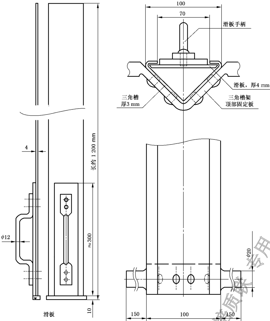
图 2 d) 三角槽形探管
