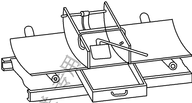
图 2 g) 停带采样框
