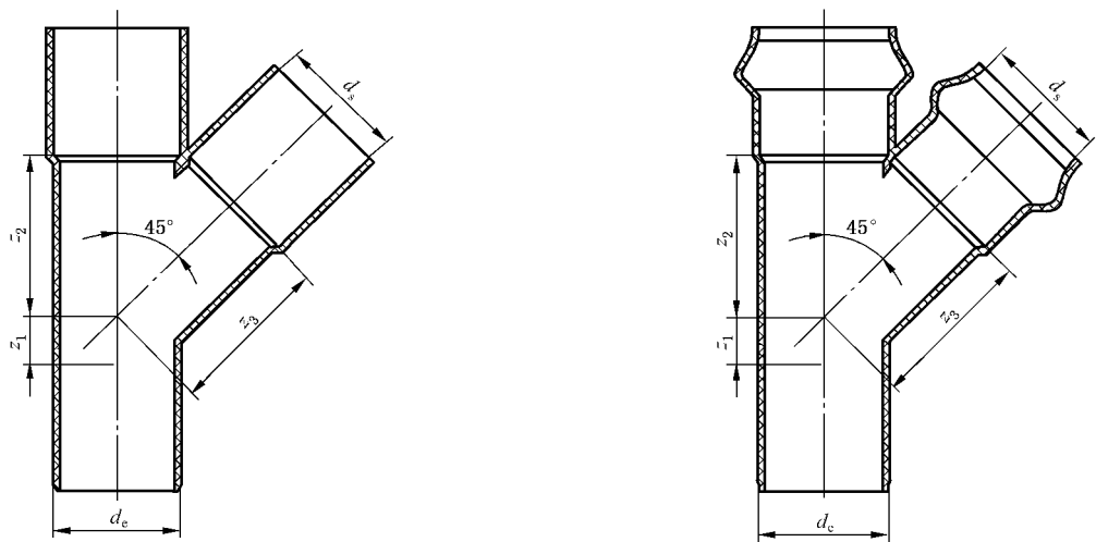
b) 45°带插口斜三通示意图
