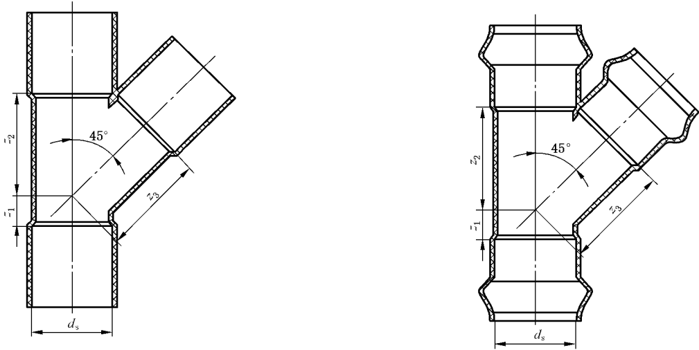
a) 45°斜三通示意图
