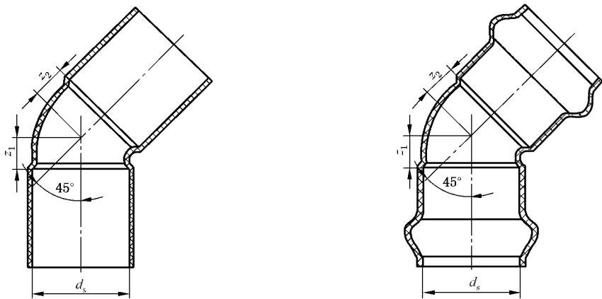
a) 45°弯头示意图
