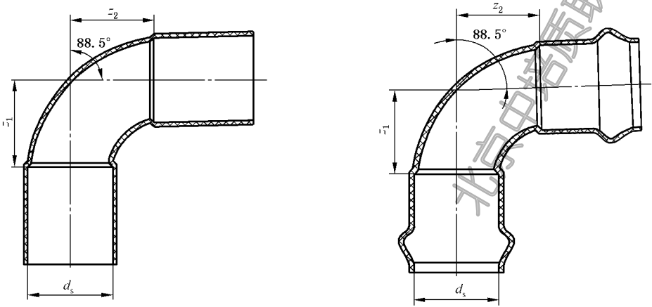
c) 90°弯头示意图
