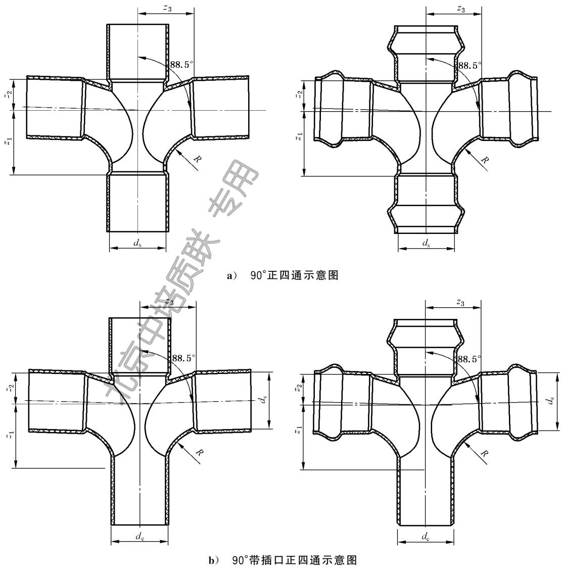
图 B.5 90°四通示意图
