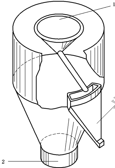
c) 旋转容器型
