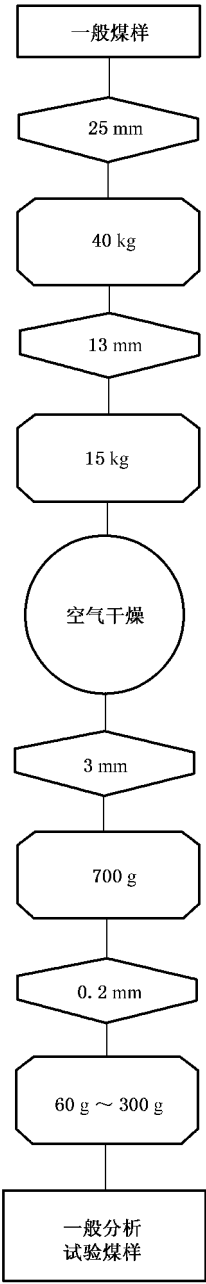
图 10 一般分析试验煤样制备程序示例
