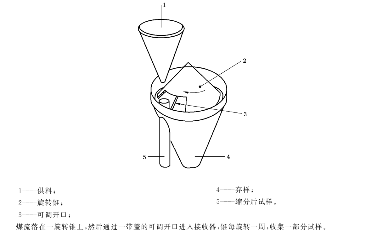
b) 旋转锥型
