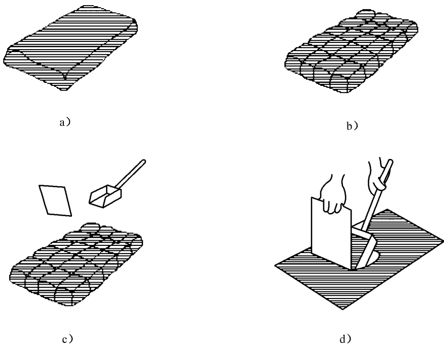
图 5 棋盘缩分法
