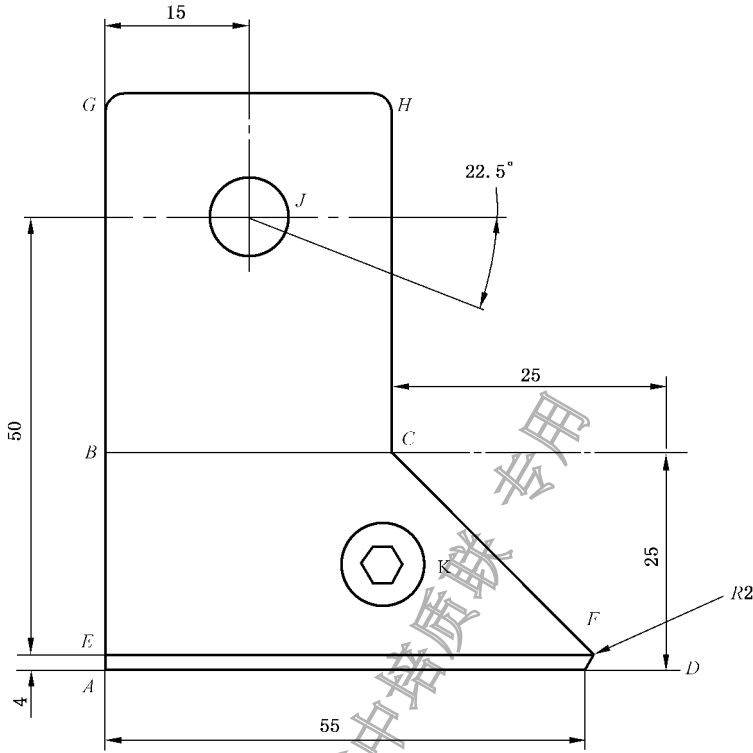
图 44 上夹具
