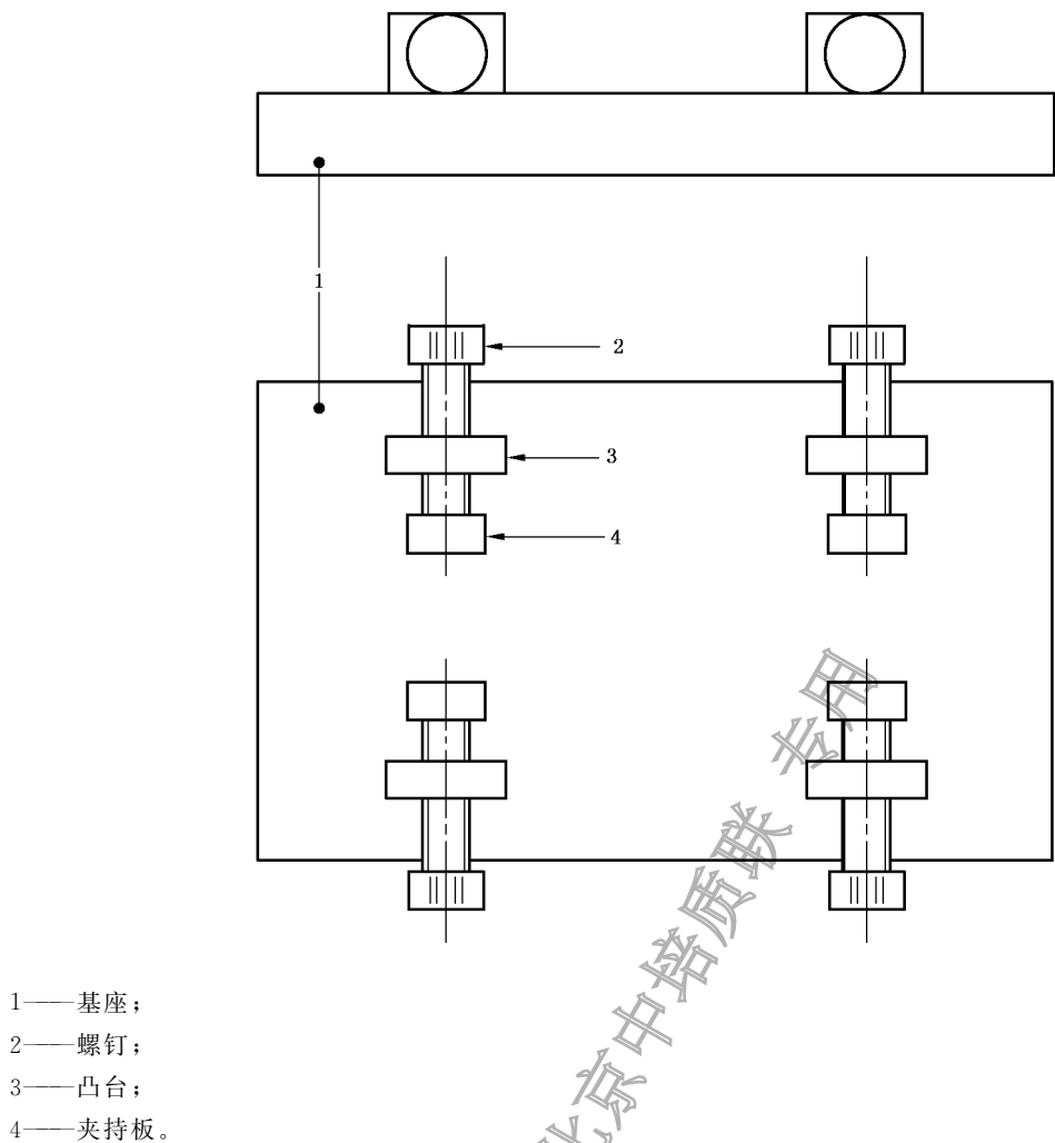
图 32 夹持装置
