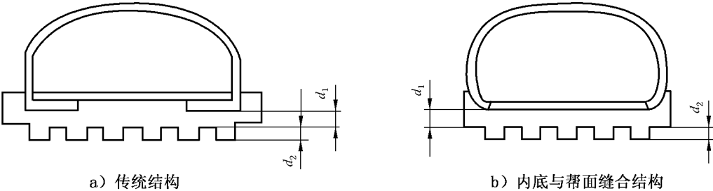
图 51 直接注压、硫化和胶粘的外底
