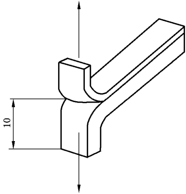
图 4 制备的试样
