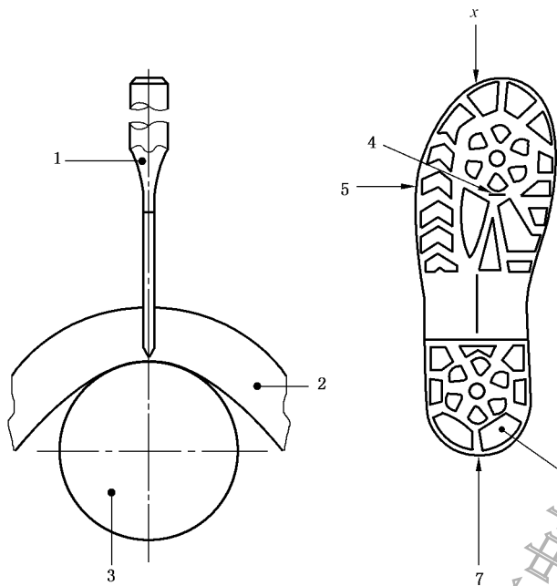
图 58 割口刀
