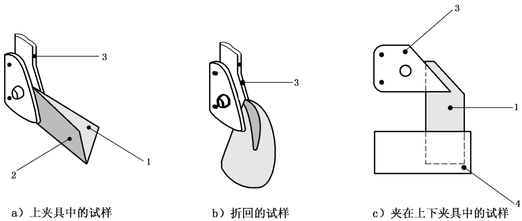
图 44 上夹具
