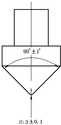
图 9 冲击锤
