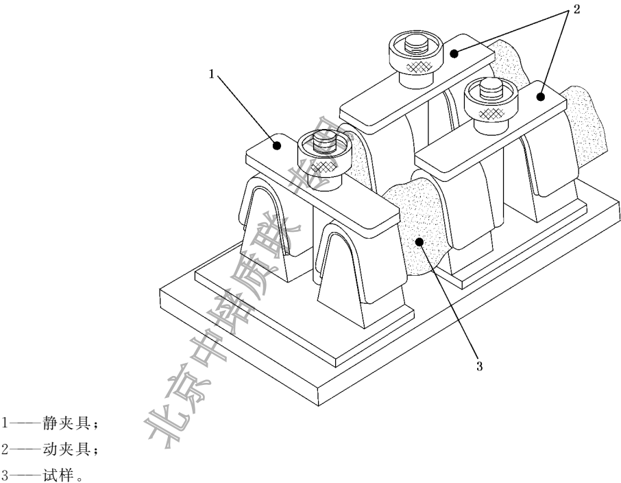
图 40 耐折装置
