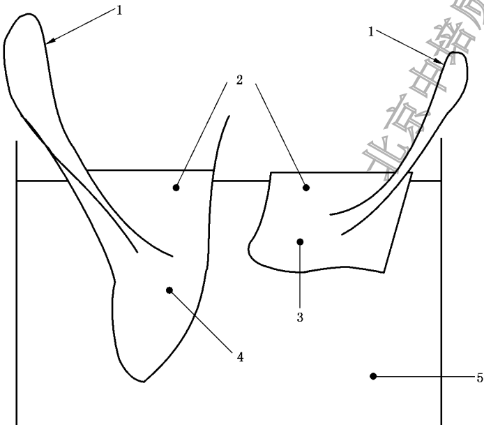
1——帮助从试样中移走的带子； 2——装满蜡的模具； 3——后跟端模具； 4——足趾端模具； 5——装砂的容器。
