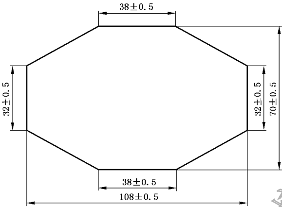
图 38 试样尺寸
