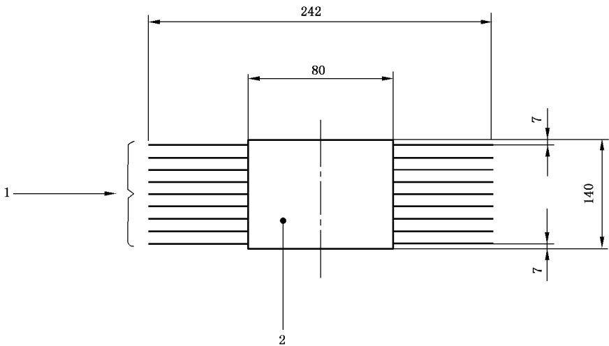
图 29 刷示意图
