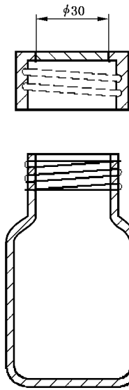
图 41 用于水蒸气渗透性测试的瓶
