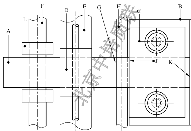
b) 试样、屈挠臂及辊轴的平面图
