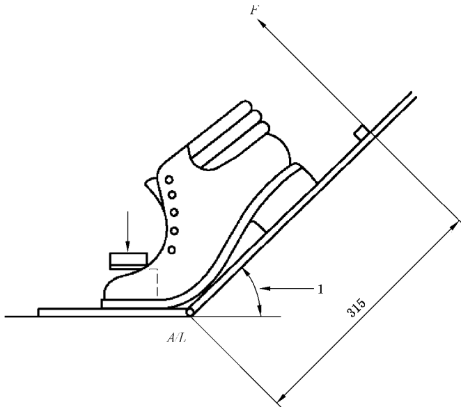
图 56 耐折角
