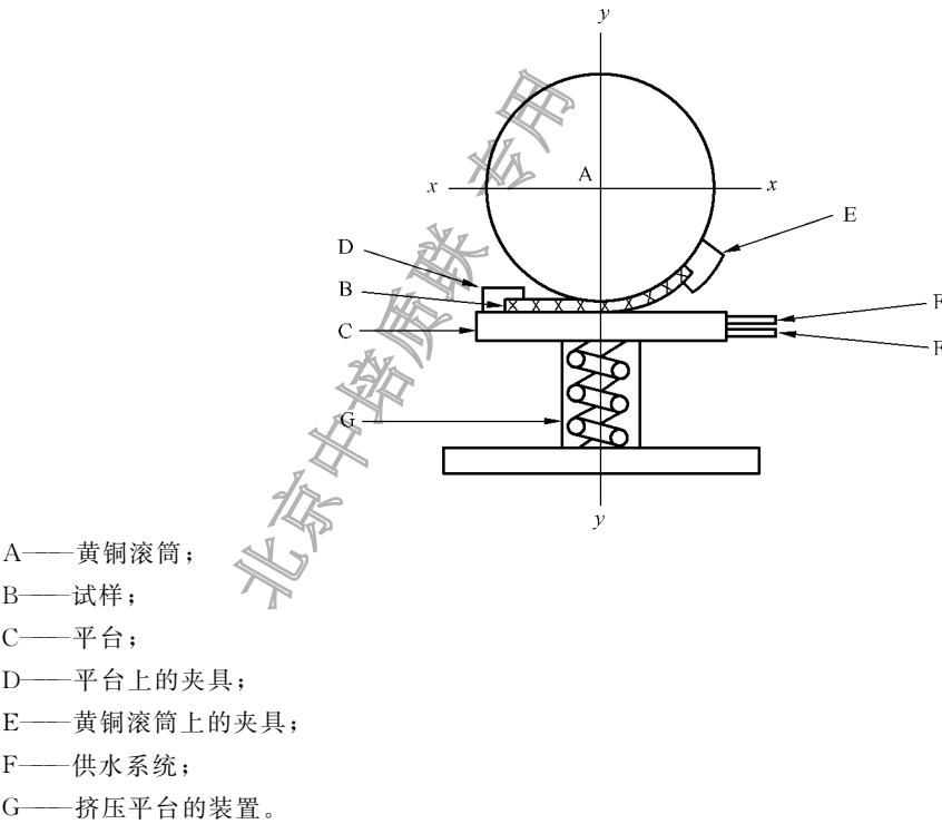
图 49 测试装置示意图
