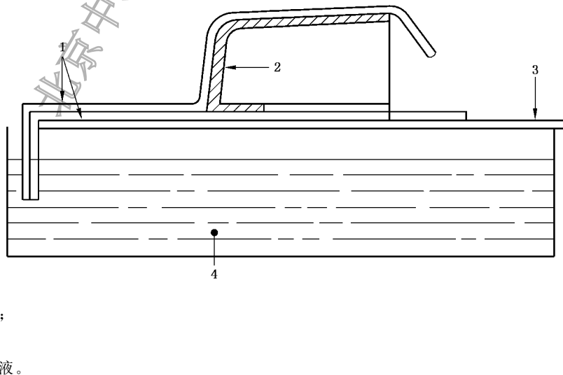
图 14 保护包头耐腐蚀性测试装置
