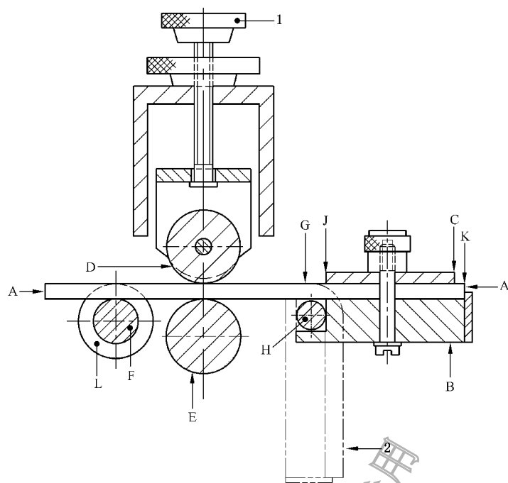
a) 试样、屈挠臂及辊轴的侧面图
