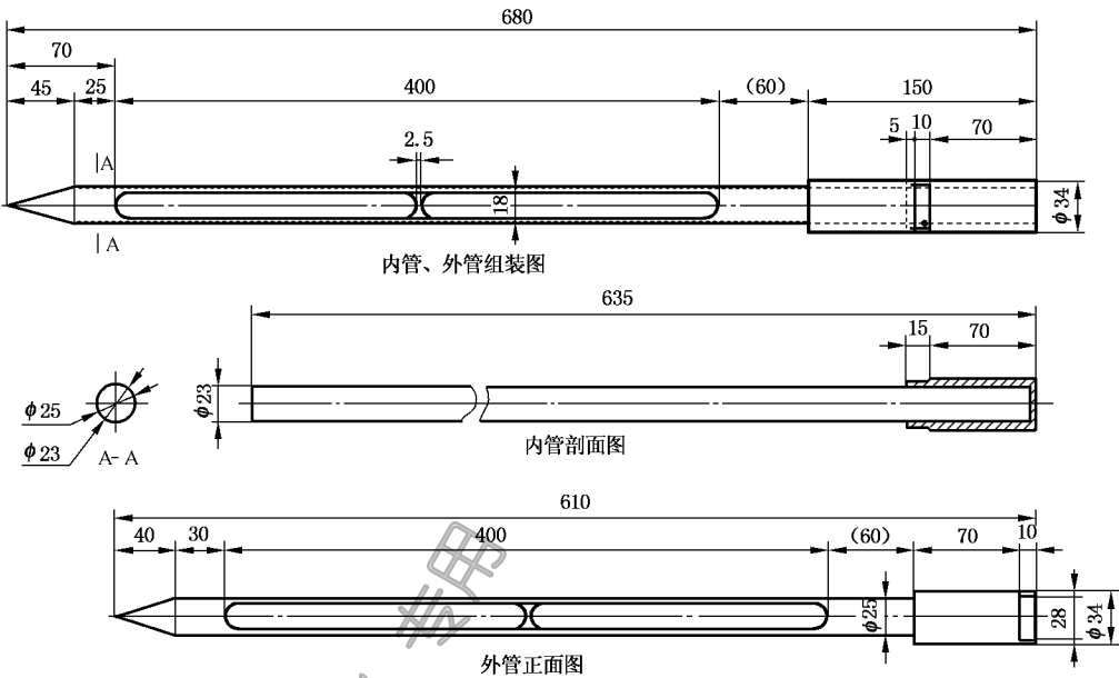
图 1 取样探子
