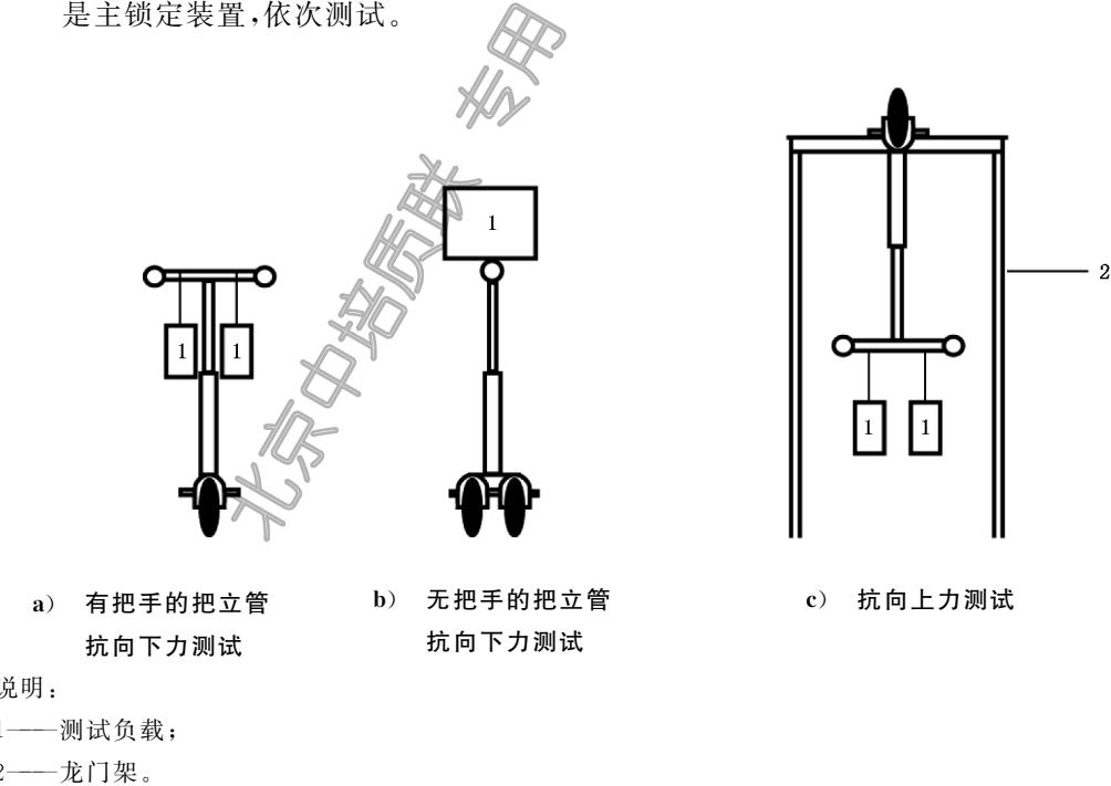
图 4 把立管测试
