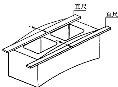
图 1 弯曲测量法
