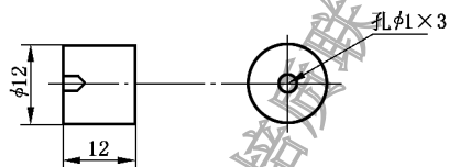
图 6 测长头
