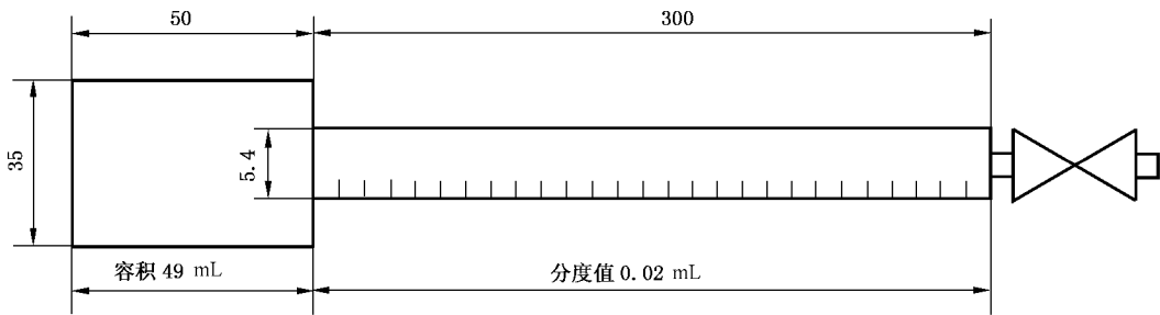
图 1 用于溶解度测定的圆筒
