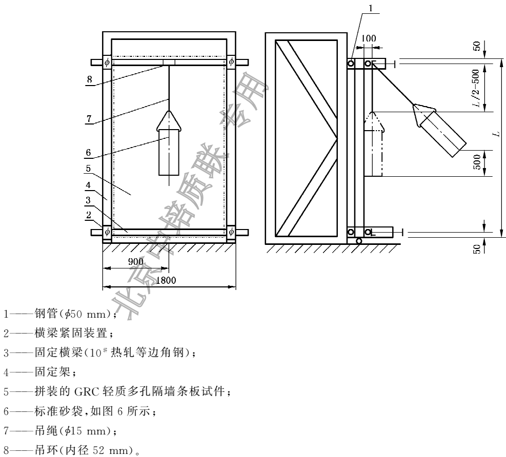
图 5 抗冲击强度的试验装置
