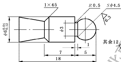
图 4 测量头
