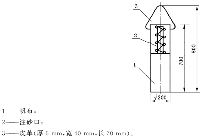
图 6 标准砂袋
