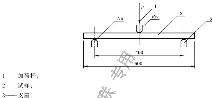
图 9 抗折破坏荷载的加荷示意图
