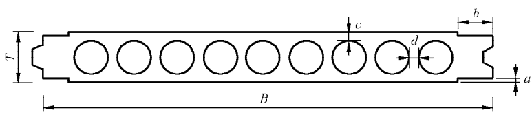
图 2 GRC 轻质多孔隔墙条板断面示意图
