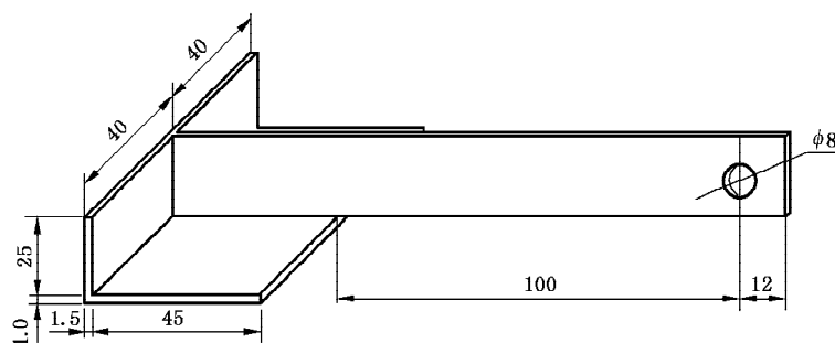
图 7 钢板吊挂件
