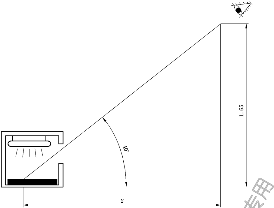
图 3 目测评价用装置
