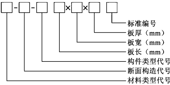
图 2 轻质条板产品型号标记示意图
